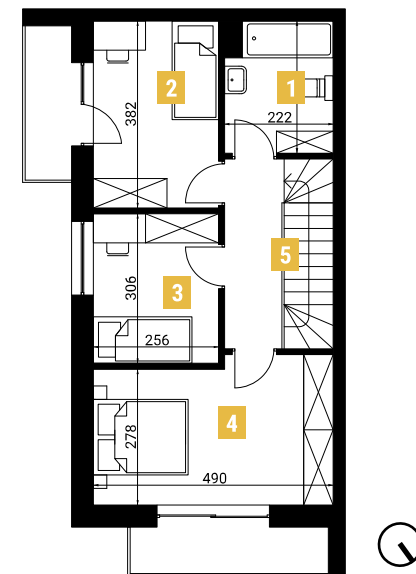
Rzut poddasza
